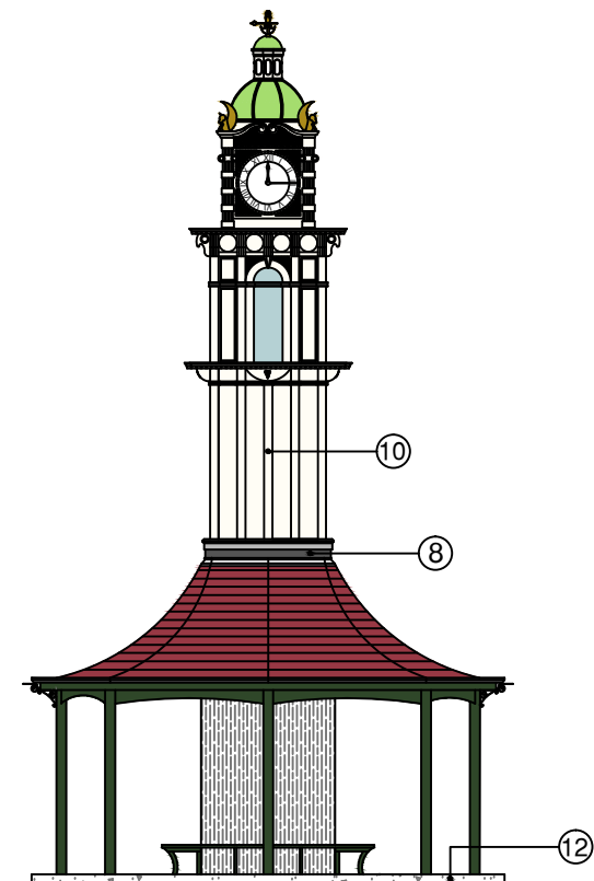
RIGHT ELEVATION
